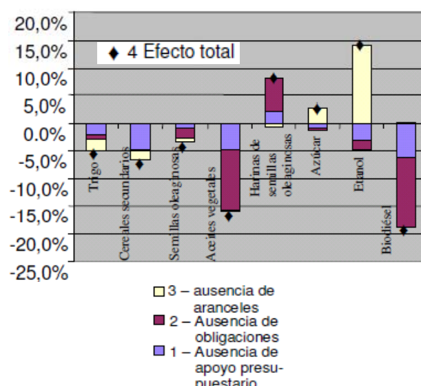
Figura 4: Impacto de la supresión del apoyo a los biocombustibles en los precios mundiales de los productos básicos
