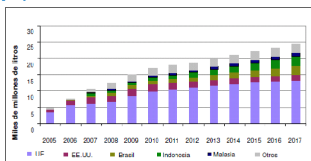
Figura 2: Principales productores de biodiésel: proyecciones hasta 2017
